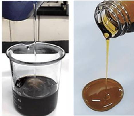
開発した低VOCの完全水溶性フェノール樹脂(右)。水で希釈しても白濁、沈殿が起こらない
